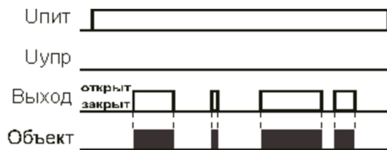
Работа выхода в режиме «dark on»
