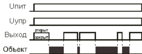
Работа выхода в режиме «dark off»
